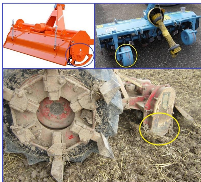
شکل ۵- تنظیم عمق کار با کفشک یا چرخ
